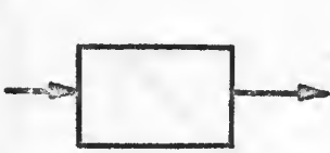
FUNKTIE
